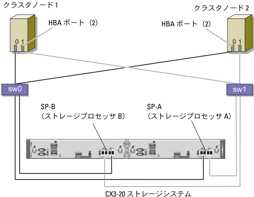
図 1-2. Del|EMC SAN 接続のファイバーチャネルクラスタのケーブル接続
